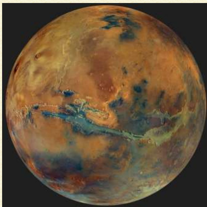
Mars
