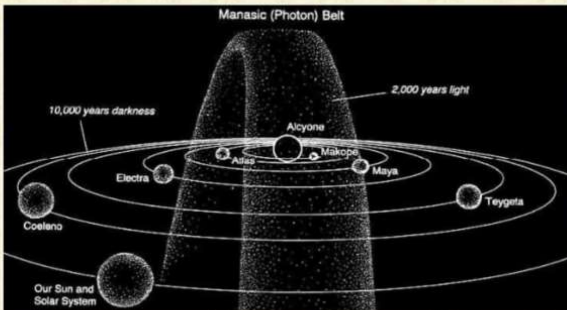
Figuur 17. Grafische afbeelding van fotonengordel . Bron Onbekend
